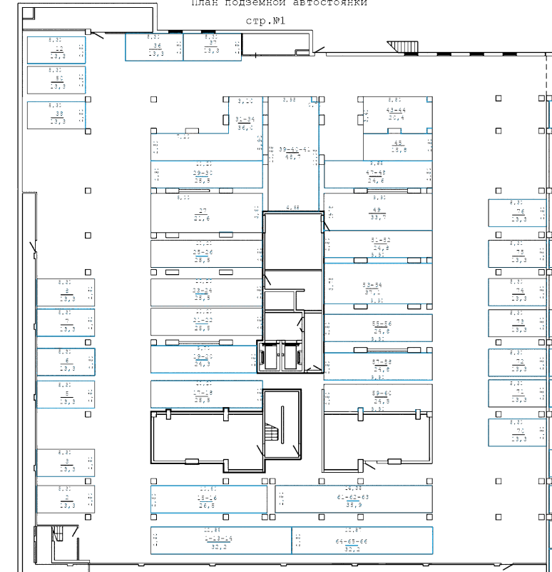
План подземной автостоянки
