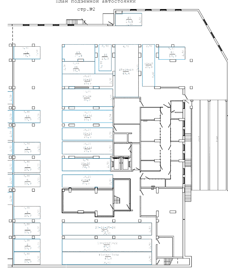
План подземной автостоянки
